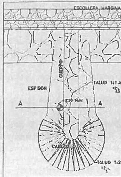
Grafico 4.46: Defensa Ribereña - Planta de Sección de Espigón de Roca
